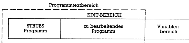
Bild 1. Struktur eines Basic-Programms und dessen Lage im Arbeitsspeicher
