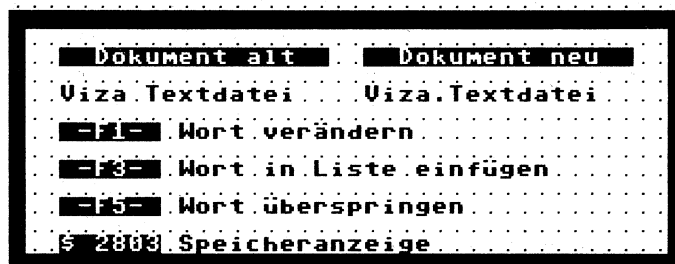
Bild 1. SPELL CHECK bei der Arbeit. Das gerade bearbeitete Wort der Textdatei befindet sich in der Mitte des Bildschirms. Die vorhergehenden Wörter finden Sie immer in der untersten Bildschirmzeile.
