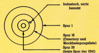
Aufzeichnungsformat einer 1541
