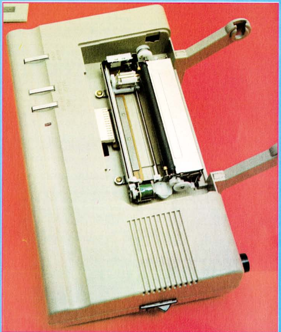
Bild 13. VC 1520. Vorne am Gerät befinden sich drei Druckschalter für Papiervorschub, Farbwechsel und für den Stiftwechsel. Vor der schwarzen Walze sieht man die Trommel mit den kleinen, metallisch glänzenden Farbkugelschreibern. Die beiden Arme an der Rückseite des Plotters nehmen die Papierrolle auf.
